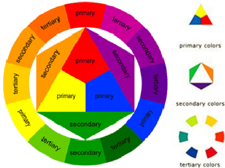
عجلة الألوان
